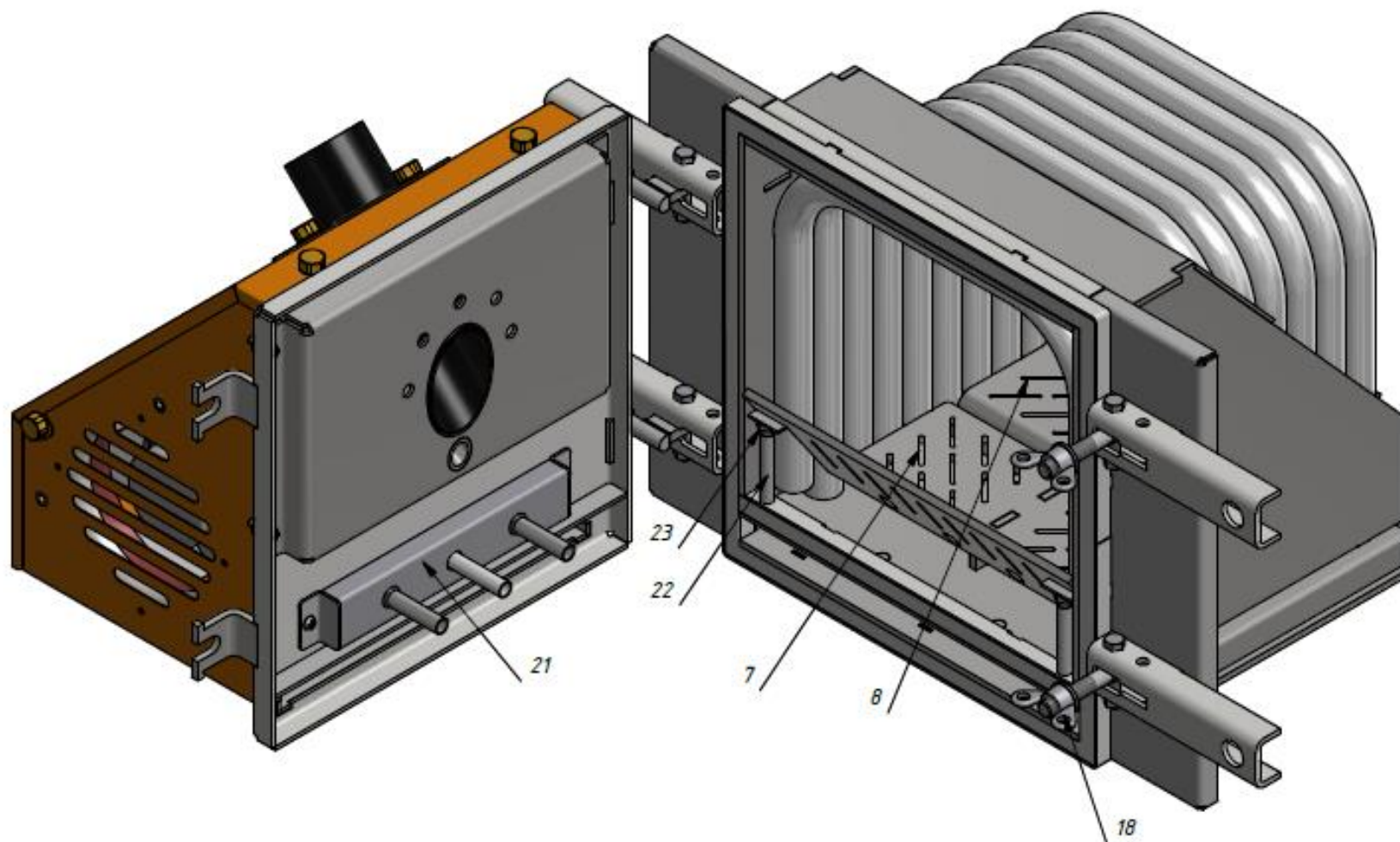
Рис.3 Горелка открытая 21-коллектор продувочный, 22 – стойка, 23 – регулировочный болт.
